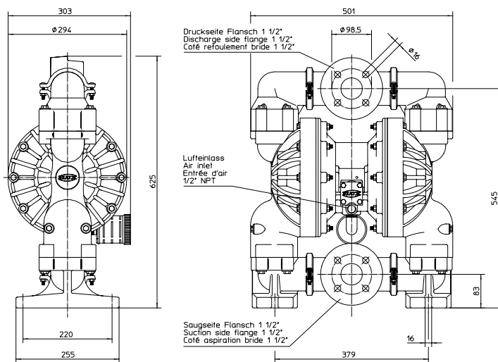
Abmessungen [mm]
