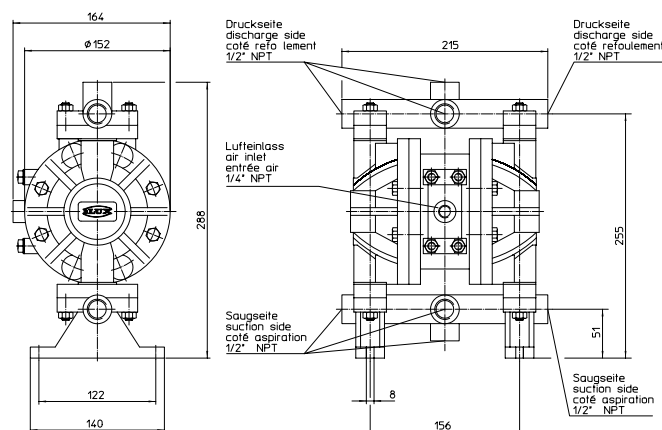
Abmessungen [mm]
