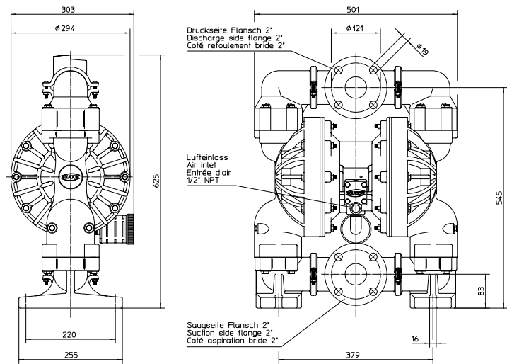
Abmessungen [mm]
