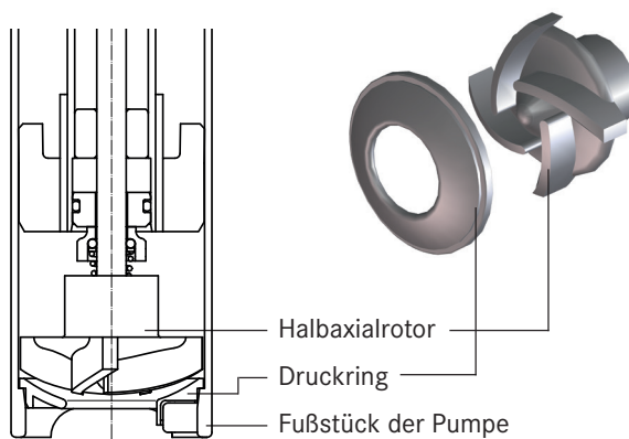
F/FP 430 mit Gleitringdichtung und Halbaxialrotor (Z-Version)
