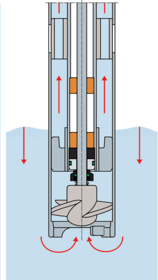
Auslauf geöffnet, Mischöffnungen geschlossen.
