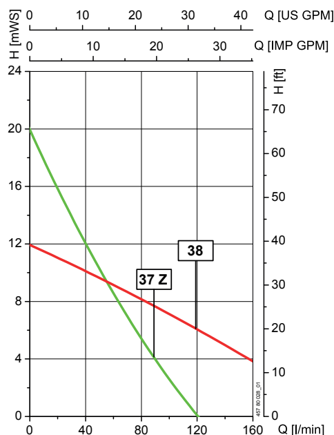
Vergleich der Kennlinien einer Fasspumpe F/FP 430 mit Antriebsmotor F 457 mit Axialrotor 38 mm und Halbaxialrotor (Z-Version) 37 mm
