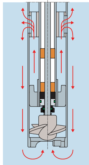
Auslauf geschlossen, Mischöffnungen geöffnet.
