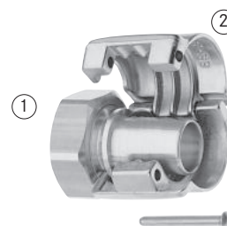
SF Ausführung mit Klemmfassung gesteckt (Spannfix)
