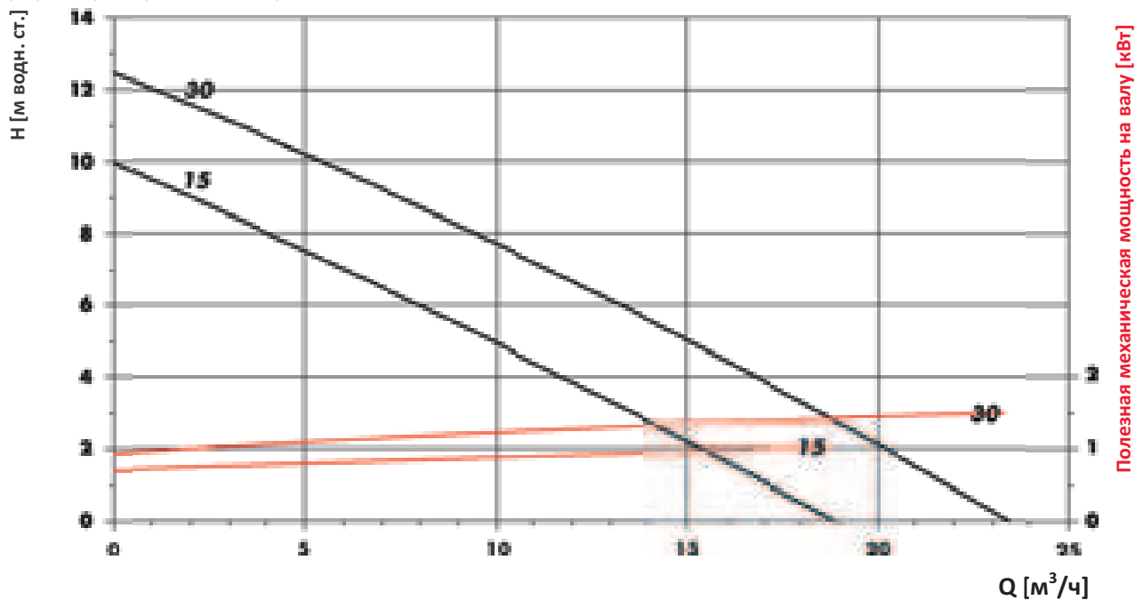
График характеристических кривых насосов FLUX моделей F 620 S-15 и F 620 S-30
