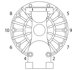
Anzugsschema Torque Sequence Couple à vérifier
