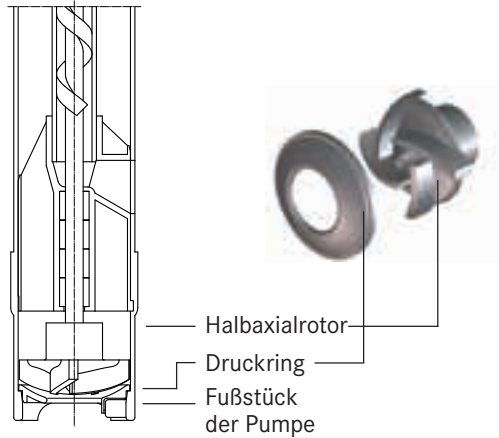
F/FP 424 mit Führungslager und Halbaxialrotor (Z-Version)
