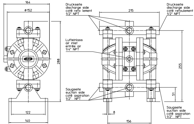
Abmessungen [mm]
