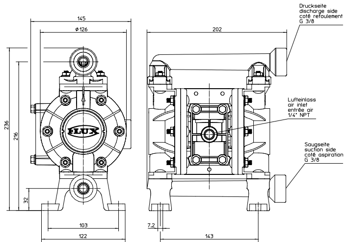
Abmessungen [mm]
