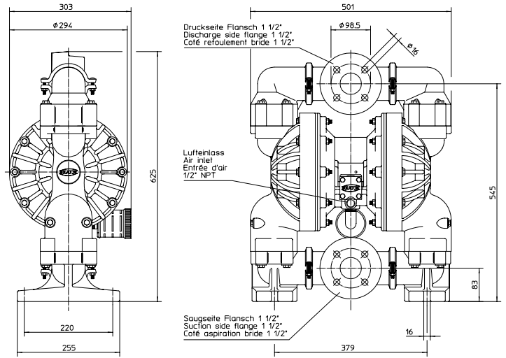
Abmessungen [mm]
