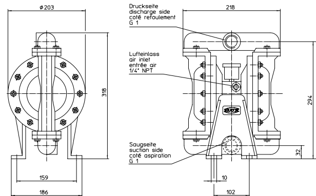
Abmessungen [mm]
