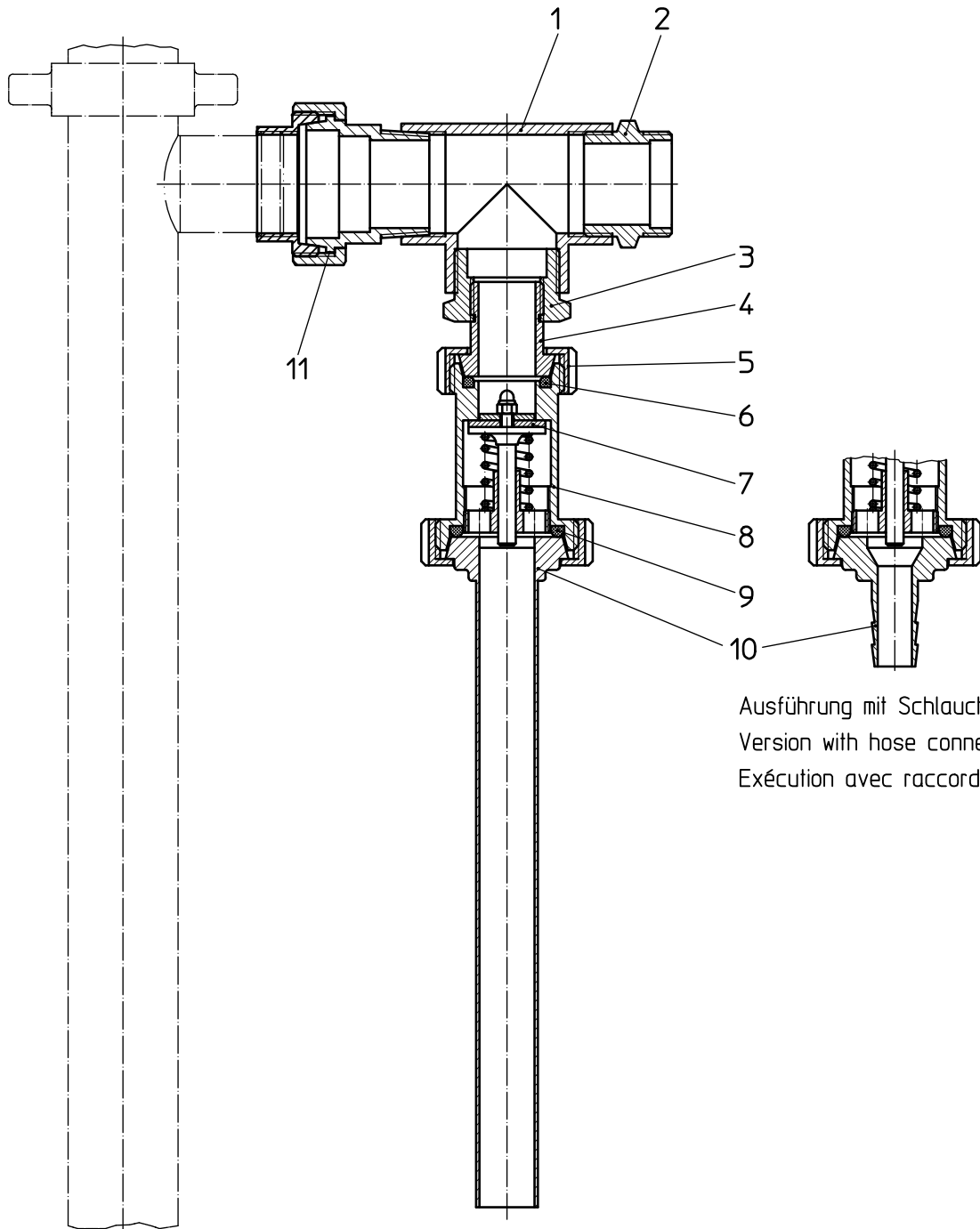
Ausführung mit Rückflussrohr Version with flow back tube Exécution avec tube de décharge
